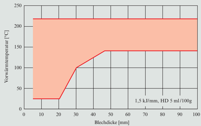
Bild 20: DILLIMAX 690: empfohlene Vorwärmtemperaturen in Abhängigkeit von der Blechdicke
