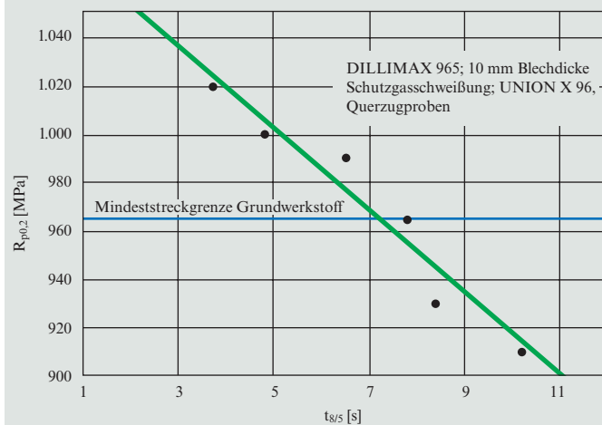
Bild 12: Auswirkungen der t_{8/5} -Zeit auf die Streckgrenze des Schweißgutes von DILLIMAX 965
