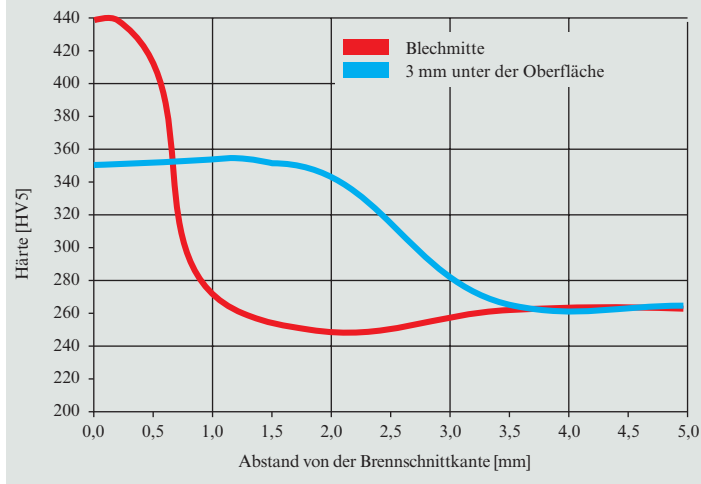
Bild 9: Typische Aufhärtung von DILLIMAX 690 an der Brennschnittkante beim Sauerstoff-Acetylen-Brennschneiden (Blechdicke: 20 bis 30 mm)
