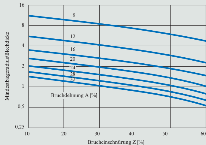
Bild 6: Mindestbiegeradien für DILLIMAX-Stähle zur Kaltumformung in Abhängigkeit von Bruchdehnung und Bruch-einschnürung
