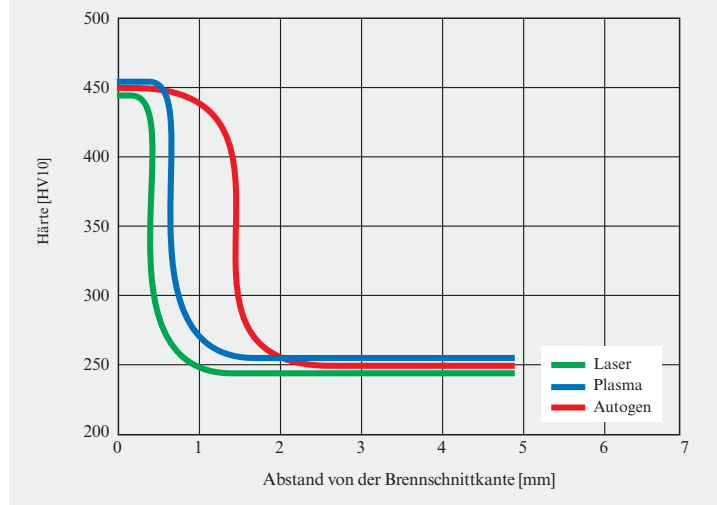
Bild 11: Typischer Einfluss von unterschiedlichen Brennschneidverfahren auf die Wärmeeinflusszone eines wasservergüteten Feinkornbaustahls mit einer Streckgrenze von 690 MPa.
