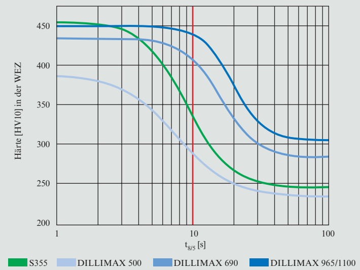
Bild 19: Aufhärtung der Wärmeeinflusszonen unterschiedlicher DILLIMAX-Stähle im Vergleich mit konventionellem S355 nach der Abkühlung mit verschiedenen t_{8/5} -Zeiten
