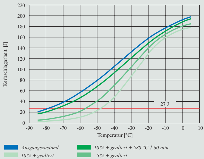
Bild 8: Typische Kerbschlagarbeit-Temperatur-Kurven eines DILLIMAX 690 T (Blechdicke 30 mm) nach Kaltumformung und künstlicher Alterung
