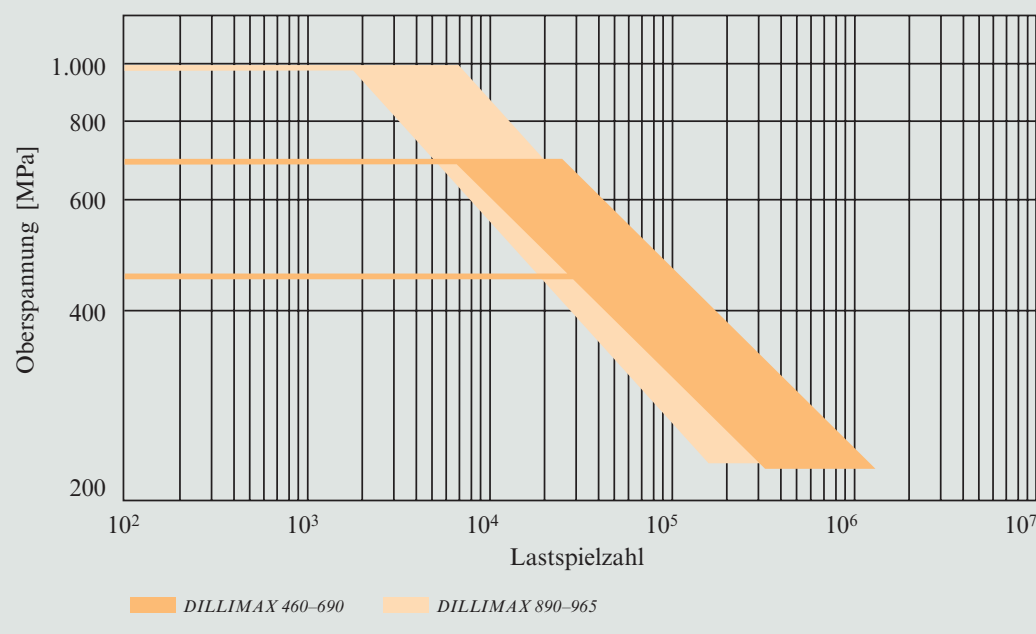
Bild 24: Wöhler-Streubänder von Schweißverbindungen aus DILLIMAX-Stählen (10 % bis 90 % Bruchwahrscheinlichkeit, V-Naht-Proben, 60°, Blechdicke 10 mm, R=0)
