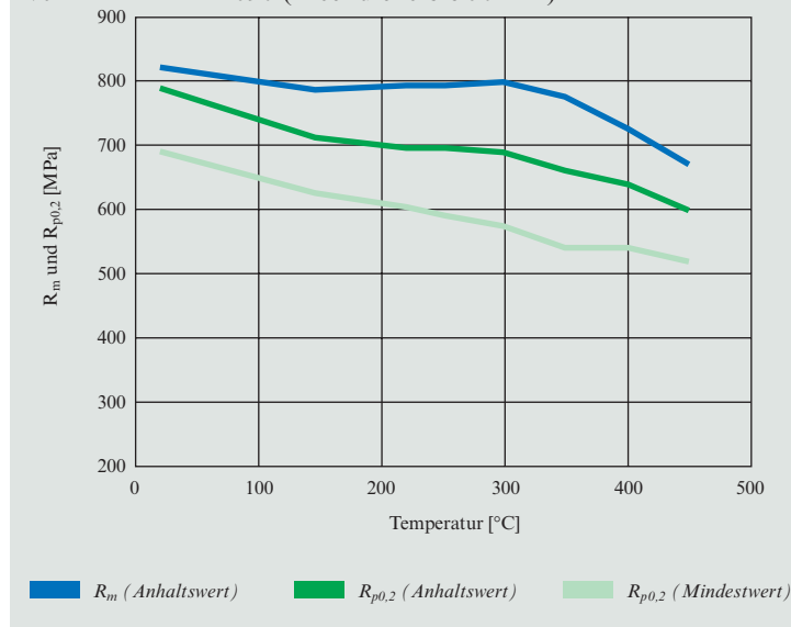
Bild 5: Einfluss der Temperatur auf die Festigkeitseigenschaften von DILLIMAX 690 (Blechdicke bis 50 mm)
