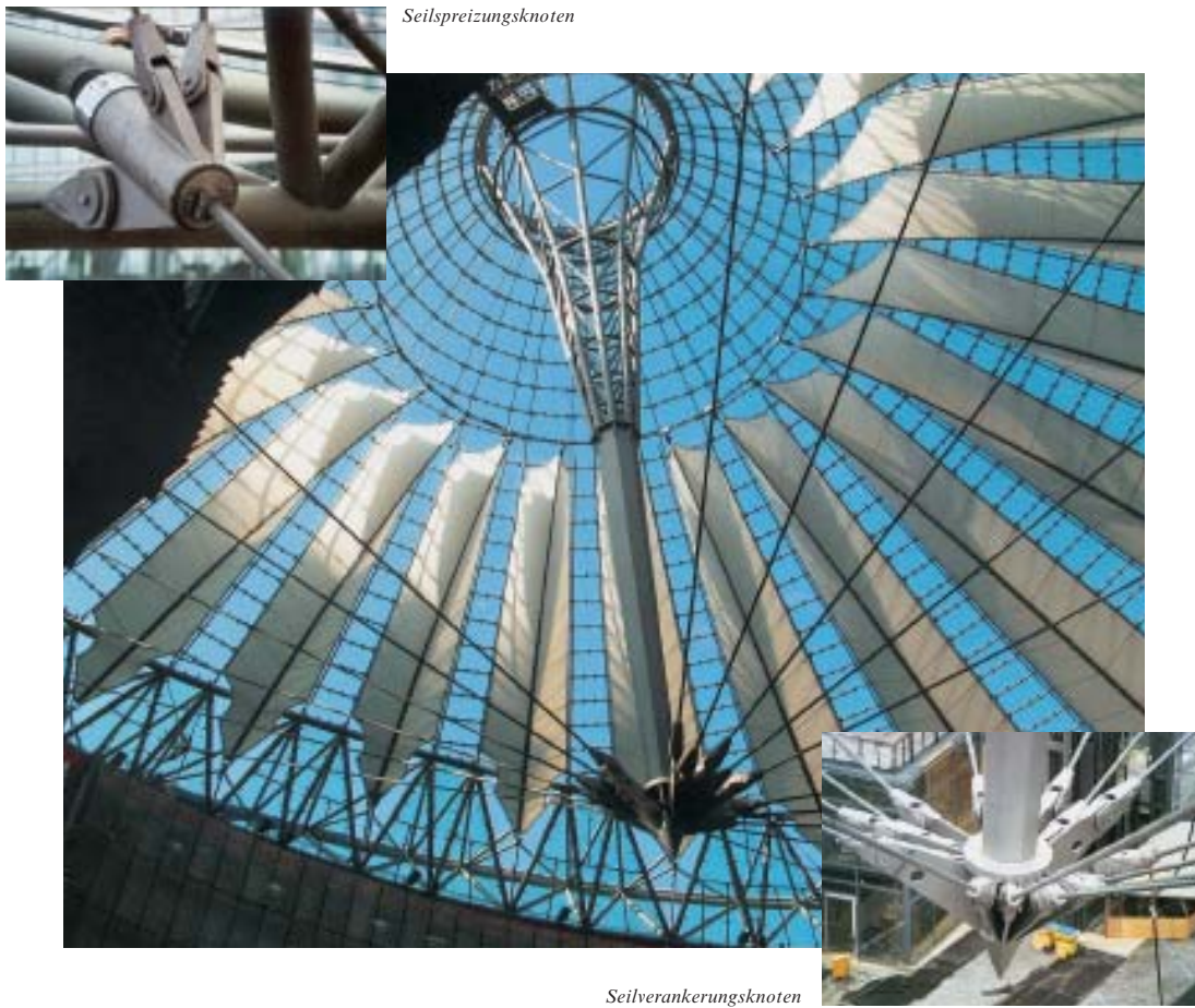
Seilverankerungsknoten
