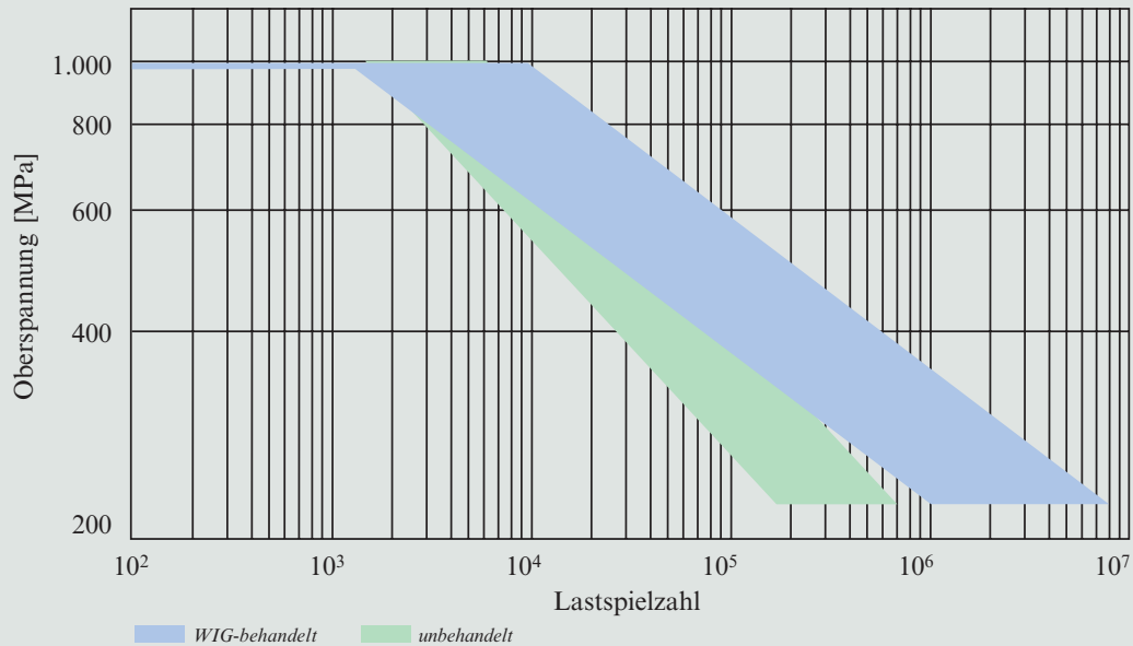
Bild 25: Einfluss einer WIG-Behandlung auf die Wöhler-Streubänder von Schweißverbindungen aus DILLIMAX 890/965 (10% bis 90% Bruchwahrscheinlichkeit, R=0)
